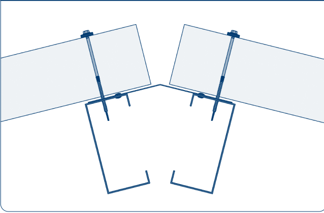
Рис. 7.111. Вид на конек крыши
