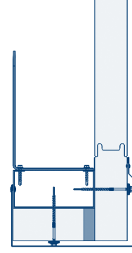
Рис. 7.128. Схема крепления горизонтального нащельника
