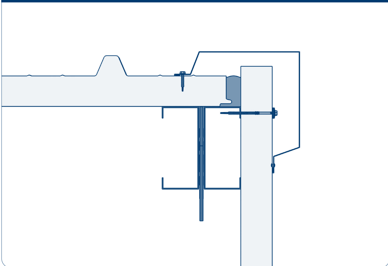
Рис. 7.140. Схема крепления нащельника
