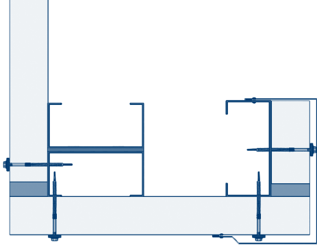
Рис. 7.127. Схема крепления вертикального нащельника
