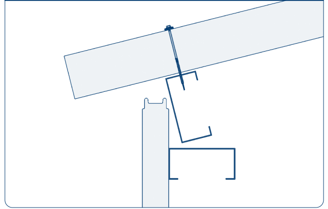
Рис. 7.112. Вид на край ската кровли
