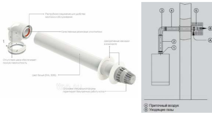
4. КОМПЛЕКТ КОАКСИАЛЬНОГО ДЫМОХОДА ROYAL THERMO 60/100 мм УНИВЕРСАЛЬНЫЙ ДЛЯ НАСТЕННЫХ КОТЛОВ ВСЕХ МАРОК
